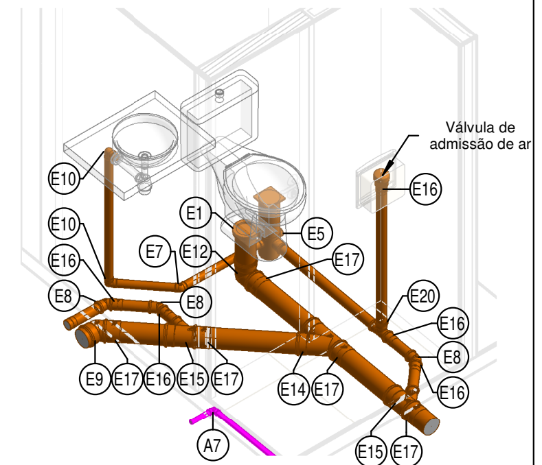
PERSPECTIVA 07 - ESGOTO
