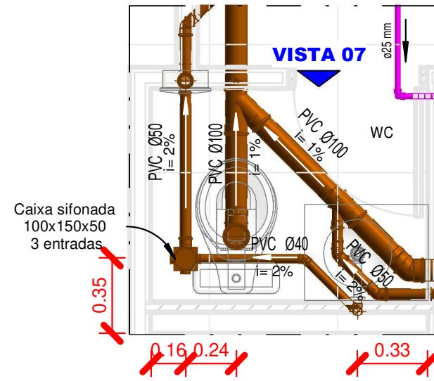
DETALHE 07 - ESGOTO 1 : 25
